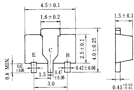
電極接続
