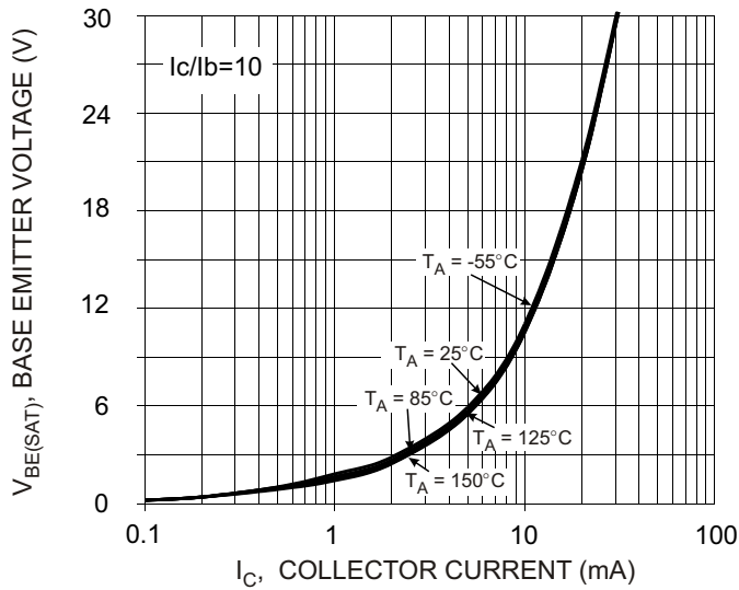
Fig. 18 V BE(SAT) vs I C
