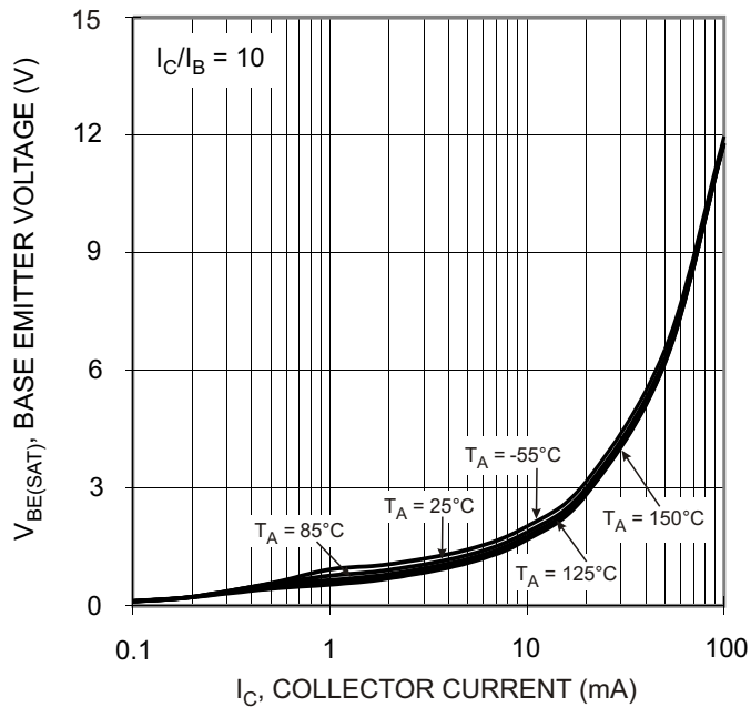
Fig. 10 V_{BE(SAT)} vs I_C
