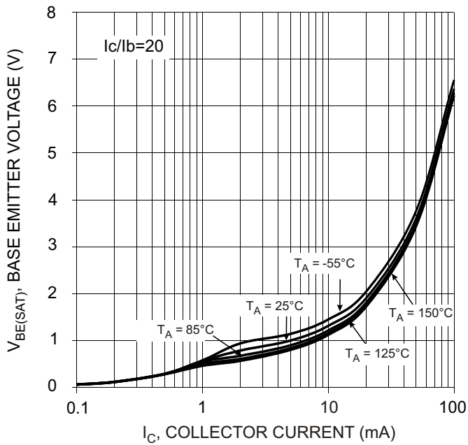
Fig. 11 V_{BE(SAT)} vs I_C
