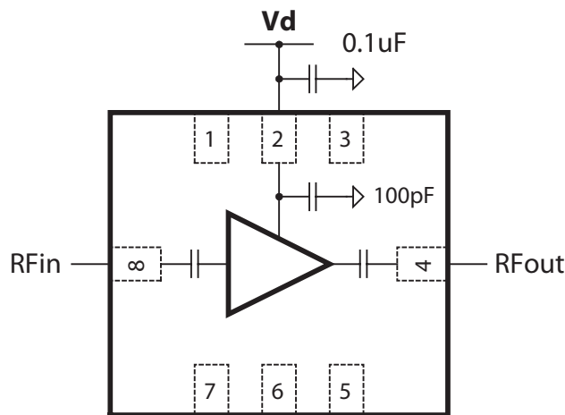
AMMP-5620
