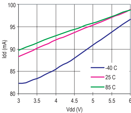
Figure 20. I dd vs. V dd
