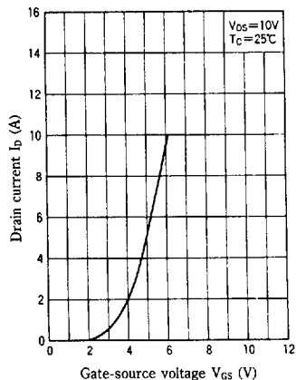
I_D - V_{GS}
