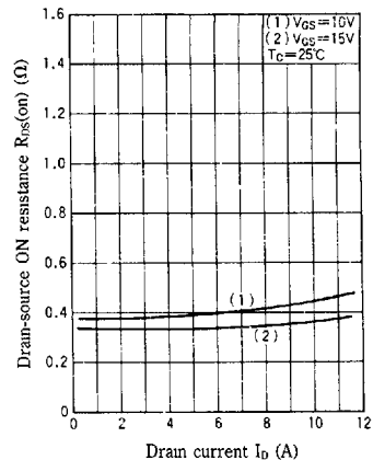
R_{DS(on)} - I_D
