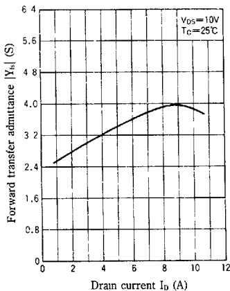
|Y_{fs}| - I_D
