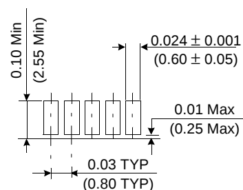
Detail Y
