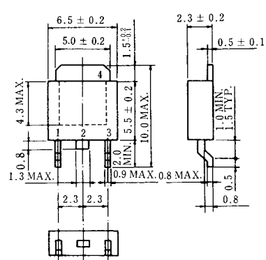
2SA1413-Z外形図
