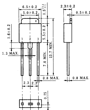
2SA1413外形図
