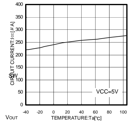
Fig.11 Ta - Icc
