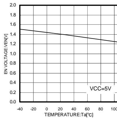
Fig.10 Ta - VEN
