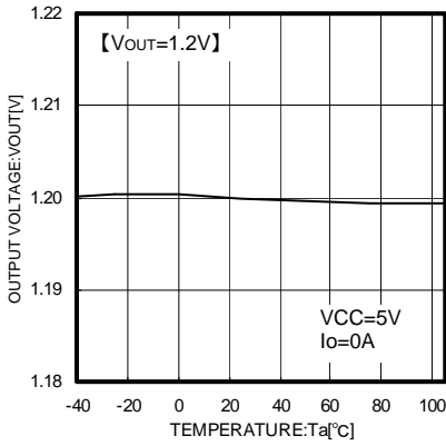
Fig. 6 Ta - VOUT
