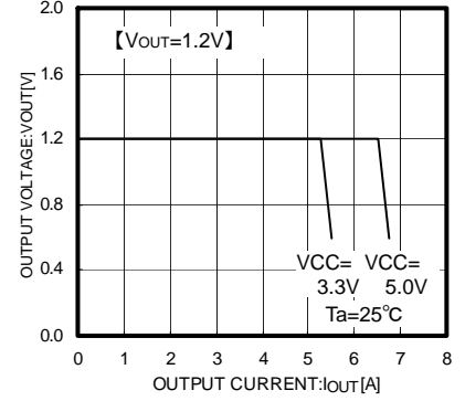
Fig.5 IOUT - VOUT
