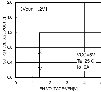
Fig.4 VEN - VOUT
