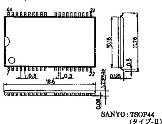
外形図 3207 (unit: mm)
