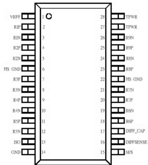
AR7519-TSSOP28
