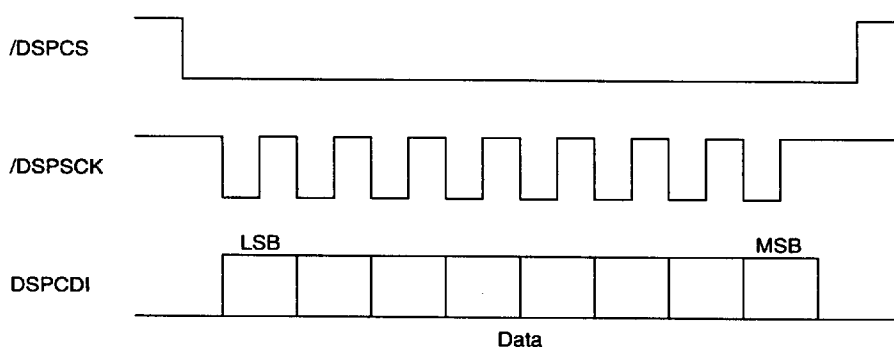
DSP Interface Format
