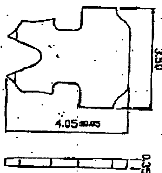
"1": 2 PRONGS FOR STRANDED WIRE 多芯線用二叉型金片
