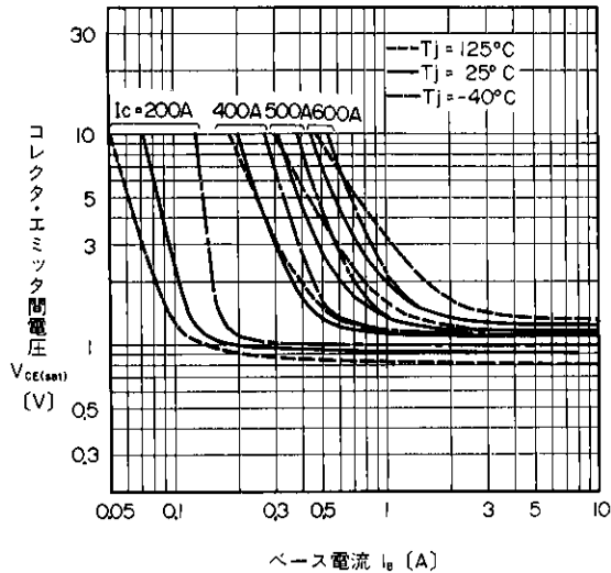
出力特性
