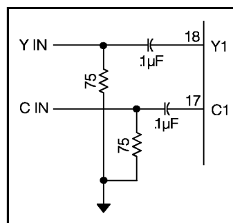
Fig. 6 - S-Video Input
