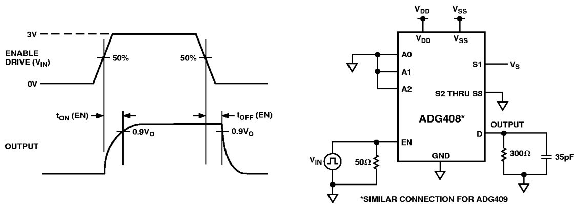
Test Circuit 7. Enable Delay, t_{ON}(EN) , t_{OFF}(EN)
