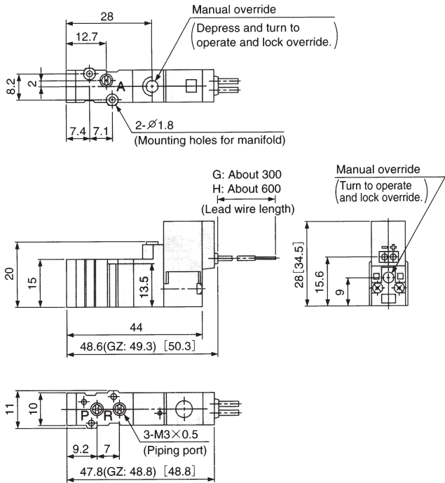
L type plug connector (L): SYJ3□2-□L□□-M3
