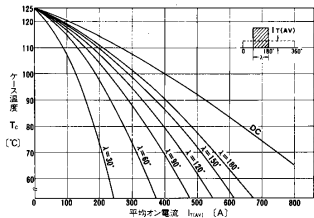
平均オン電流—ケース温度(方形波電流)
