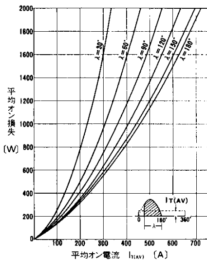
平均オン損失(正弦波電流)
