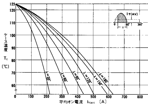
平均オン電流—ケース温度(正弦波電流)
