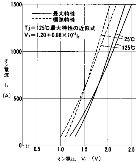
オン電圧特性
