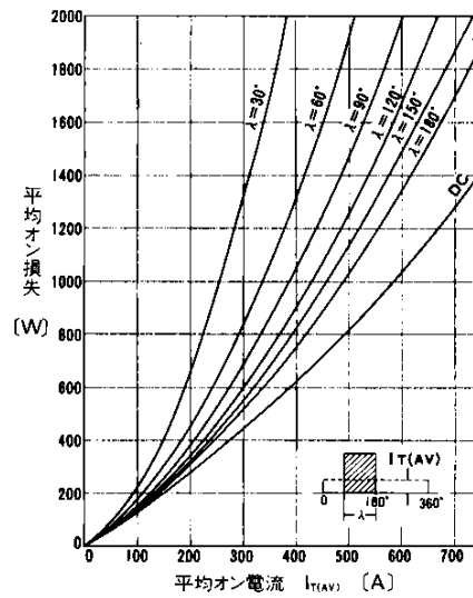
平均オン損失(方形波電流)
