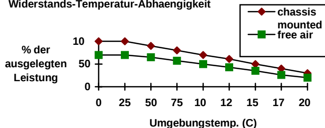
Widerstands-Temperatur-Abhängigkeit
