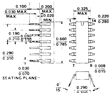
AD530D TO-116
