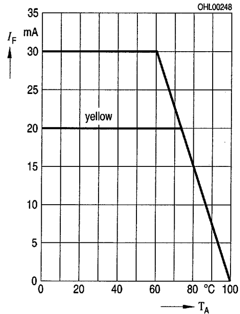
Maximal zulässiger Durchlaßstrom Max. permissible forward current I_F = f(T_A)
