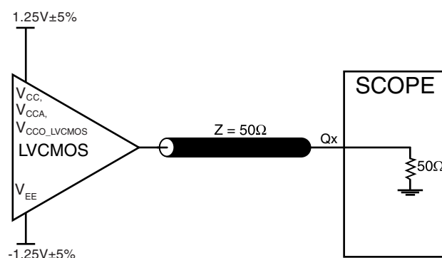
2.5V LVCMOS OUTPUT LOAD AC TEST CIRCUIT
