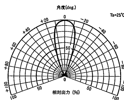
■指向特性
