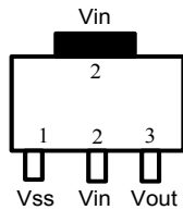
SOT-223 (N)
