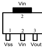
SOT-89 (R)
