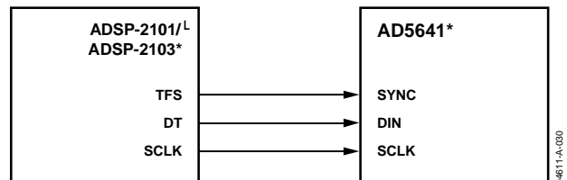
Figure 29. AD5641 to ADSP-2101/ADSP-2103 Interface
