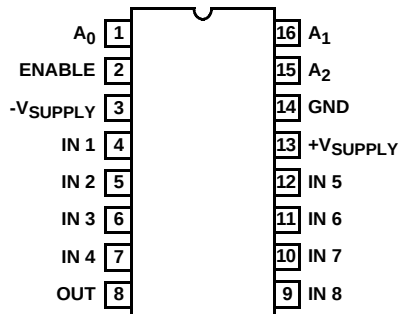
HI-548 (CERDIP, PDIP, SOIC)
