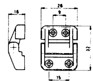
Hinge PA 22039
