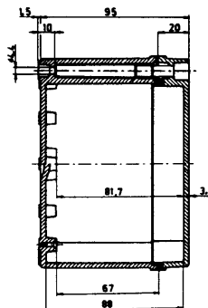
Fastening lug type II FP 22040
