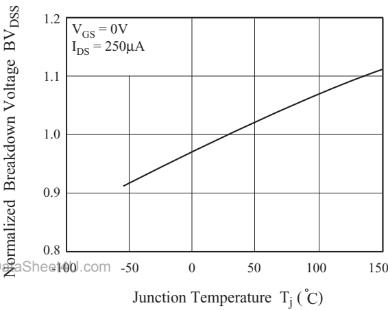
Fig4. BV_{DSS} - T_j
