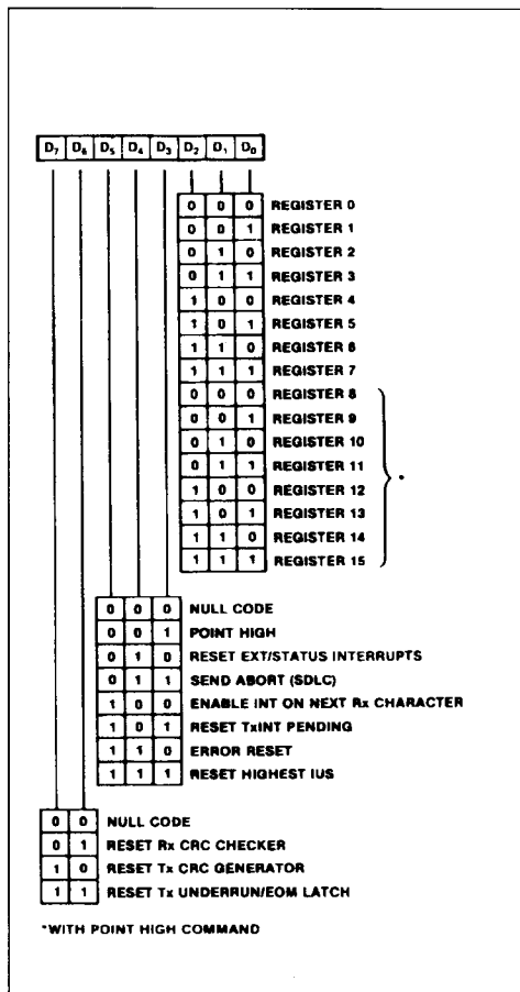
Figure 43 : Write Register 0 (Z8530).
