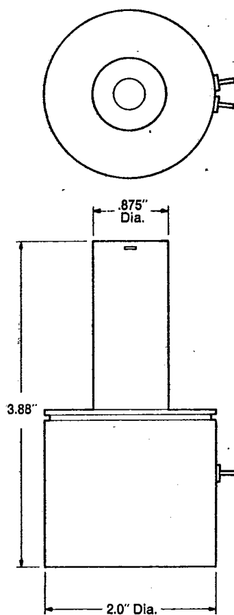
Fig. 8 — Dewar type D04EJ.
