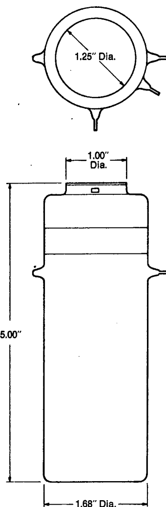
Fig. 9 — Dewar type D05E.
