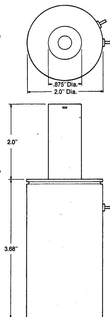
Fig. 10 — Dewar type D06EJ.
