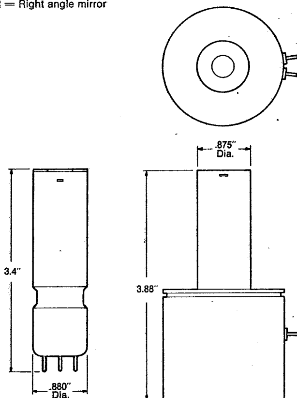
Fig. 7 Dewar type D03E.
