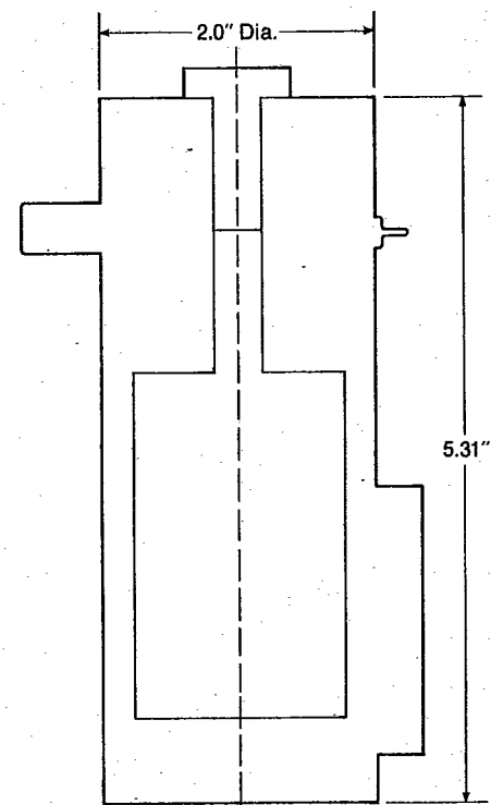
Fig. 15 — Dewar type D155S.
