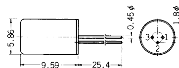
外形図-28
