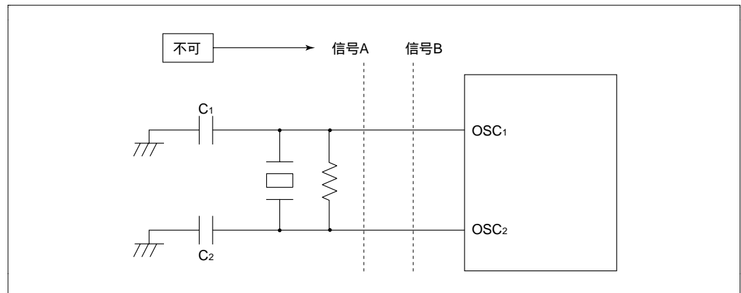
図 4.5 発振回路部のボード設計に関する注意事項
