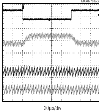
D0 DYNAMIC VID CODE CHANGE
