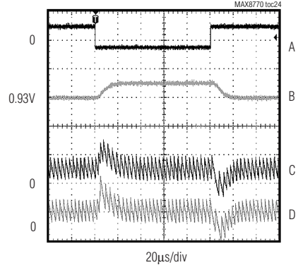
D3 DYNAMIC VID CODE CHANGE
