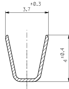
SECT.B-B
