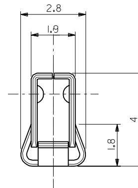
SECT.A-A
