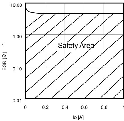
Fig.17 ESR condenser
