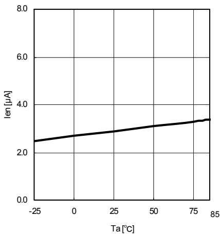
Fig.10 Ta-IEN
