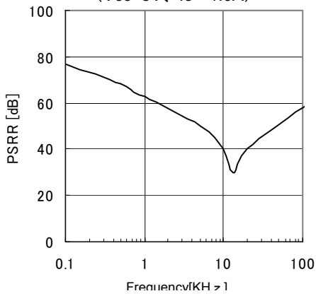
Fig.19 PSRR(Io=0mA)
