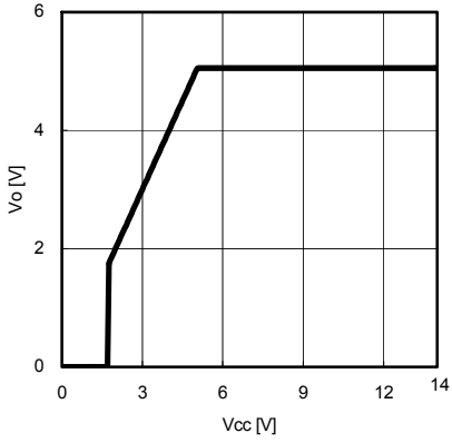
Fig.13 Vcc-Vo (Io=0mA)
