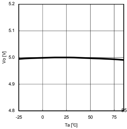
Fig.7 Ta-Vo (Io=0mA)
