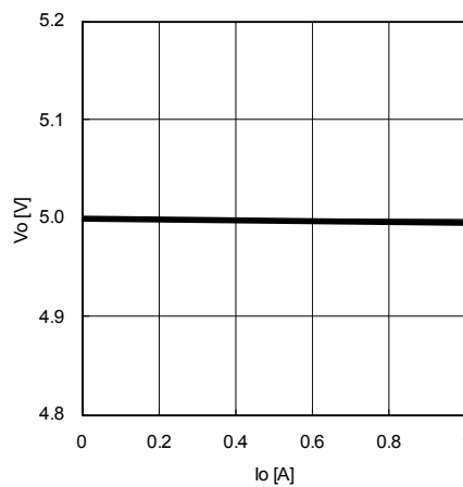
Fig.11 Io-Vo
