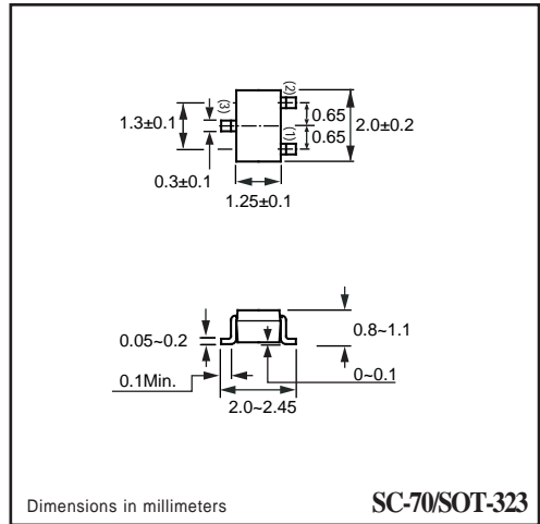
SC-70/SOT-323
