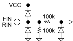
Fig.44 FIN / RIN
