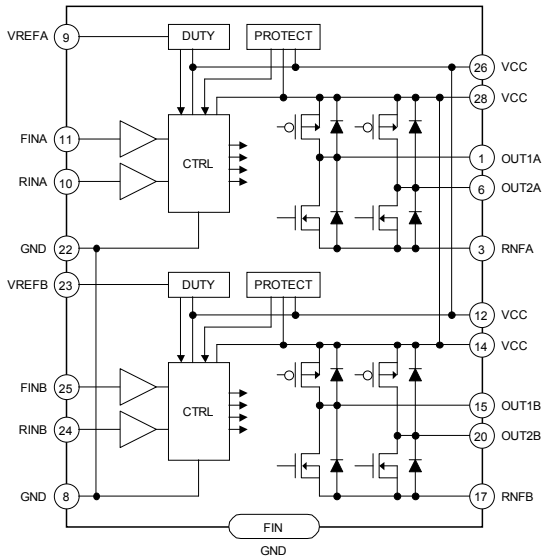
Fig.33 BD6226FM
