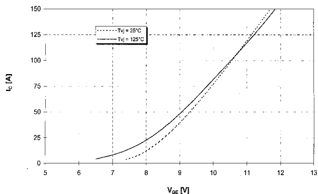
Übertragungscharakteristik (typisch) Transfer characteristic (typical)
