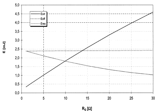
Schaltverluste (typisch) Switching losses (typical)
