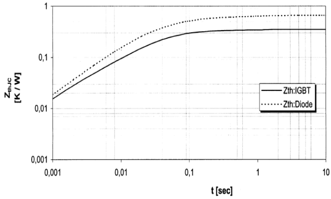
Transienter Wärmewiderstand Transient thermal impedance
