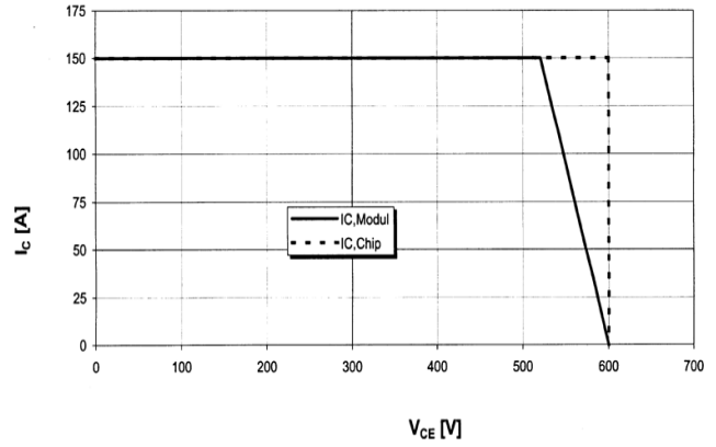
Sicherer Arbeitsbereich (RBSOA) Reverse bias safe operation area (RBSOA) V_{GE} = +15V, R_{\theta,CH} = 3,0\Omega, T_J = 125^\circ C
