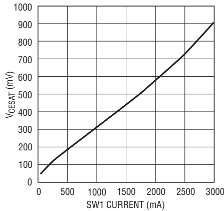
SW1 V_{\text{CESAT}}
