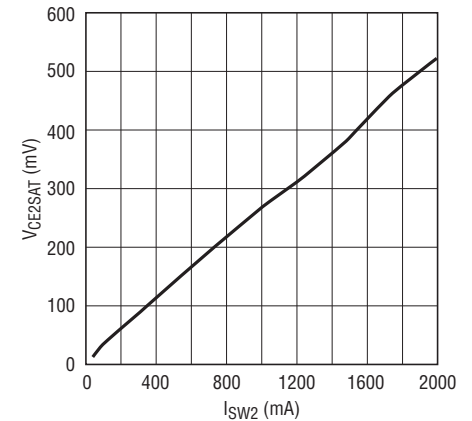
SW2 V_{\text{CESAT}}
