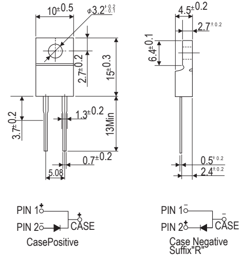
ITO-220A
