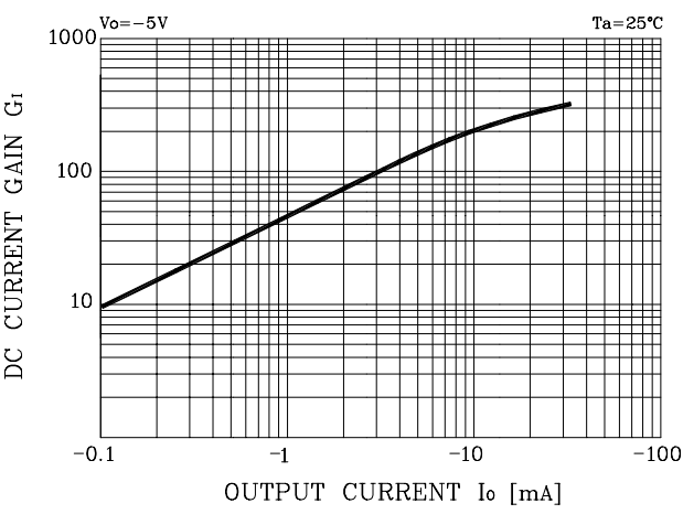
Fig. 3 G_I - I_O
