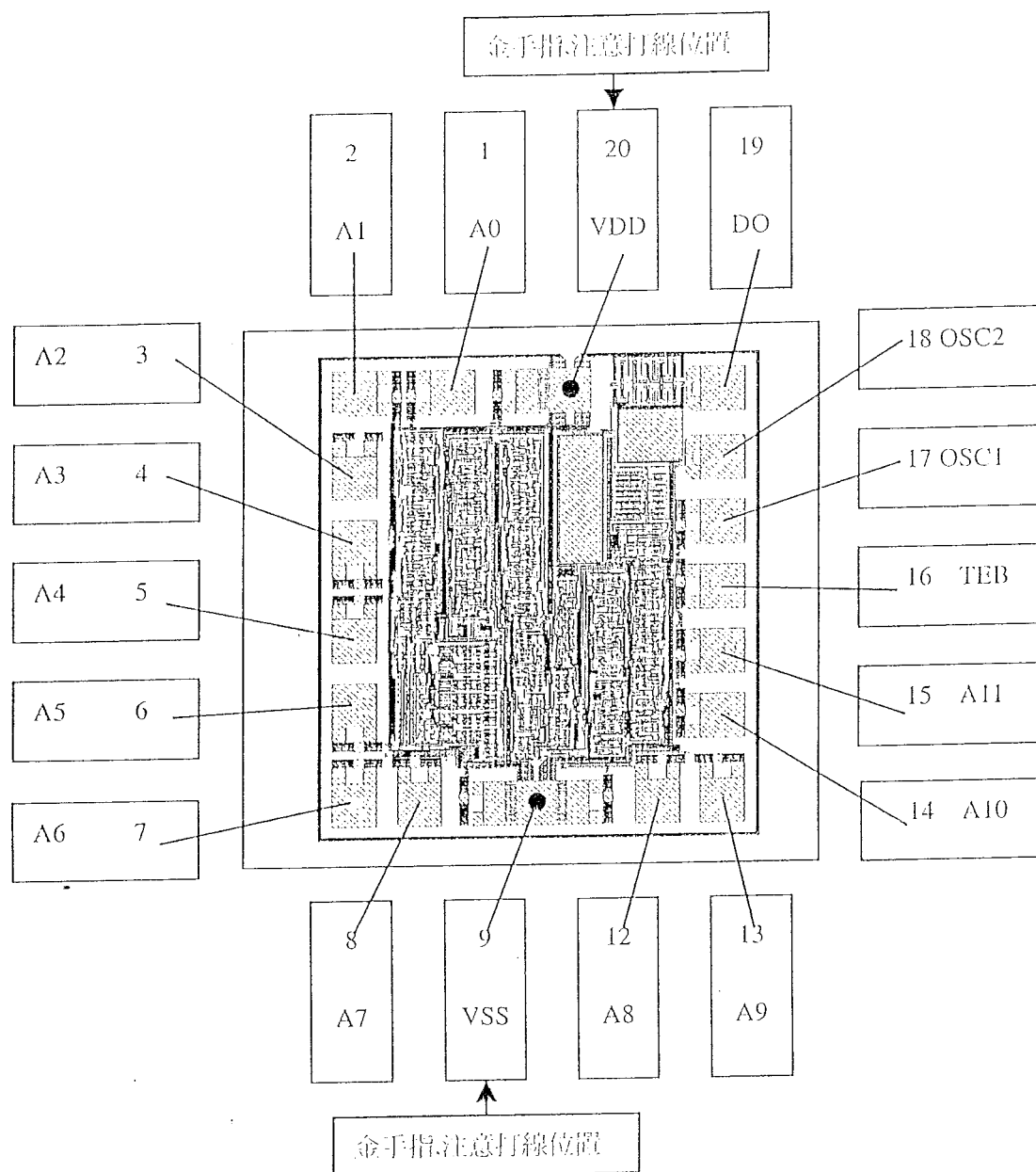
DIP-18P封装打线图
