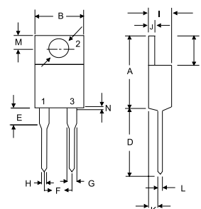
TO-220A
