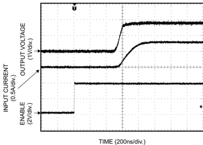
Turn-On
