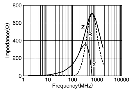
MZA2010D121C
