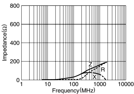
MZA2010D330C
