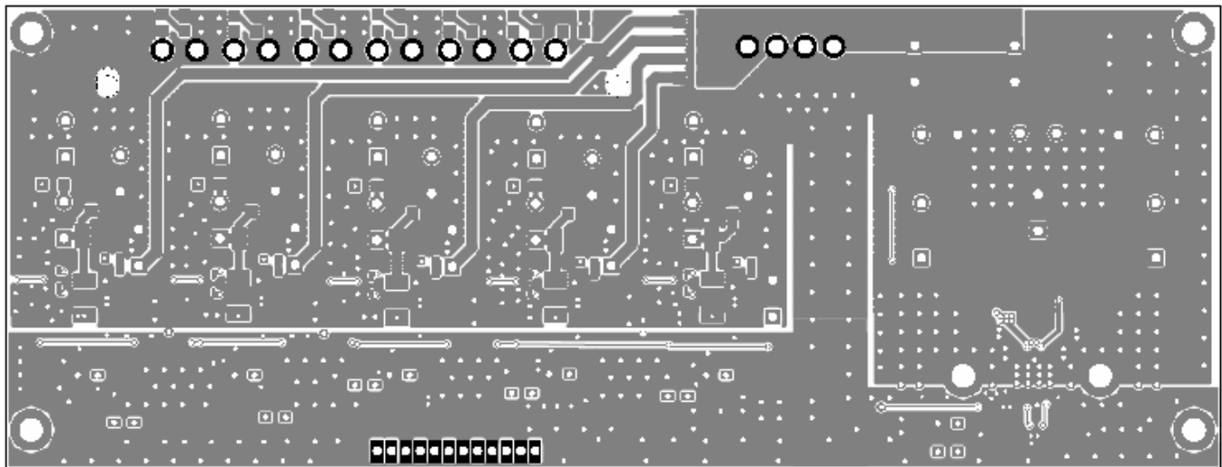
Figure 4—Bottom Layer
