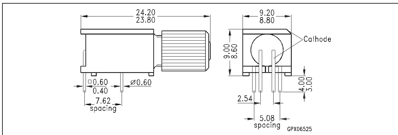
SFH 756V
