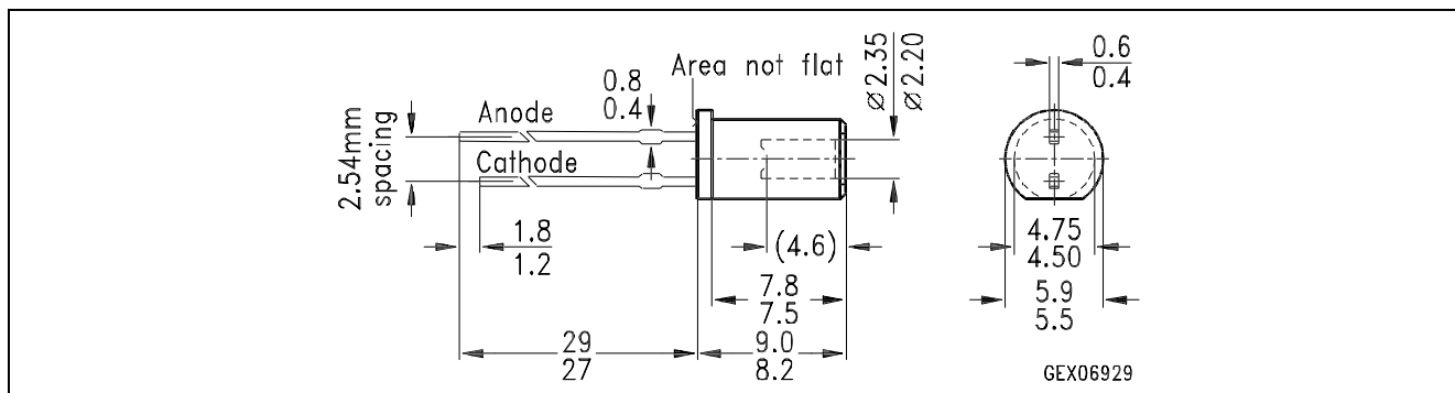
SFH 756
