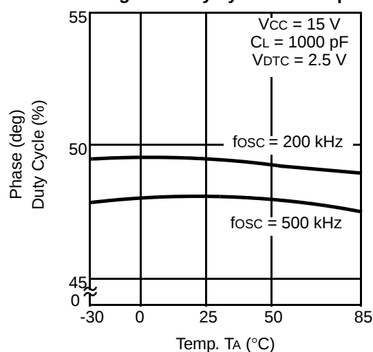
Fig. 35 -Duty cycle vs. Temp.
