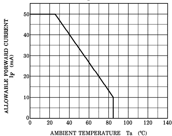
I_F - T_a
