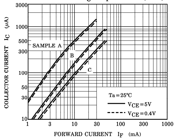
I_C - I_F (TYP.)
