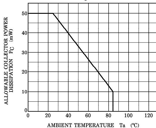
P_C - T_a
