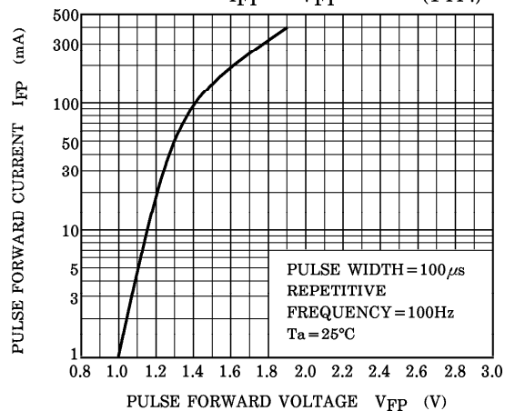
I_{FP} - V_{FP} (TYP.)
