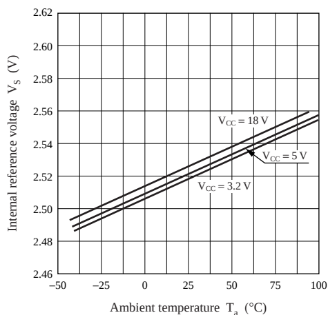
V_S - T_a
