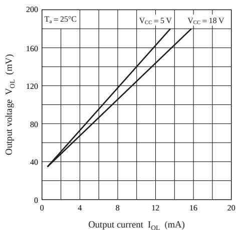
V_{OL} - I_{OL}
