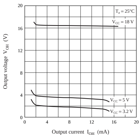
V_{OH} - I_{OH}
