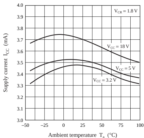
I_{CC} - T_a
