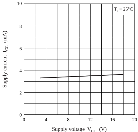
I_{CC} - V_{CC}
