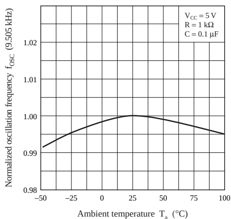
f_{OSC} - T_a
