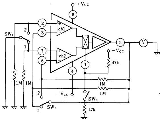
(2) I_B , I_O
