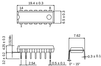
DIP14
